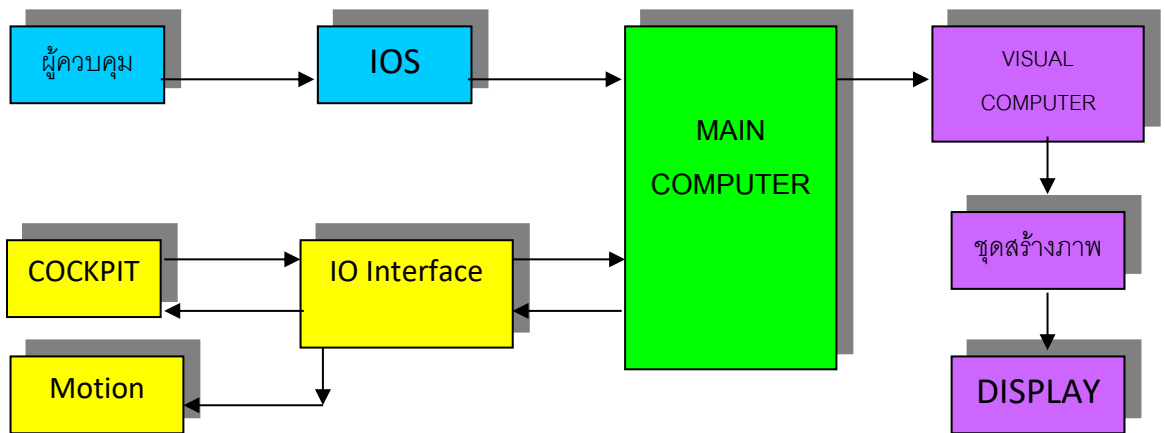
ภาพที่ ๑-๒๓ แสดง แผนผังแสดงหลักการทำงานของเครื่องฝึกบินจำลอง
