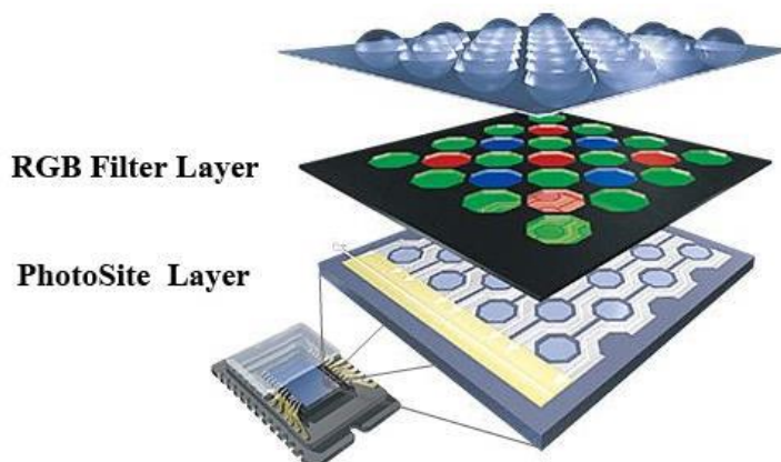
ภาพที่ ๓-๓๒ แสดงลักษณะชั้นการวางตัวของฟิลเตอร์เพื่อแยกสีที่เข้ามา
