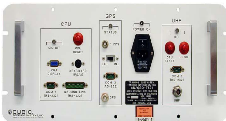
ภาพที่ ๑-๕ แสดง Surface Instrumentation Subsystem
