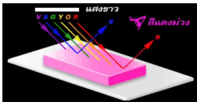
ภาพที่ ๓-๔ แสดง วัตถุสะท้อนแสงสีน้ำเงินสีแดงมากเข้าสู่เลนส์ตา ทำให้เรามองเห็นวัตถุเป็นสีแดงม่วง ที่มา : http://physicsworld.nanacity.com/physicsworld/lesson/light8.htm
