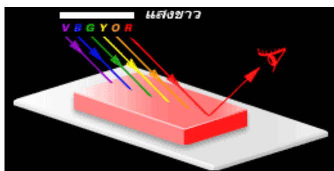
ภาพที่ ๓-๒ แสดง วัตถุสะท้อนแสงสีแดงเข้าสู่เนยน์ตา ทำให้เรามองเห็นวัตถุเป็นสีแดง
